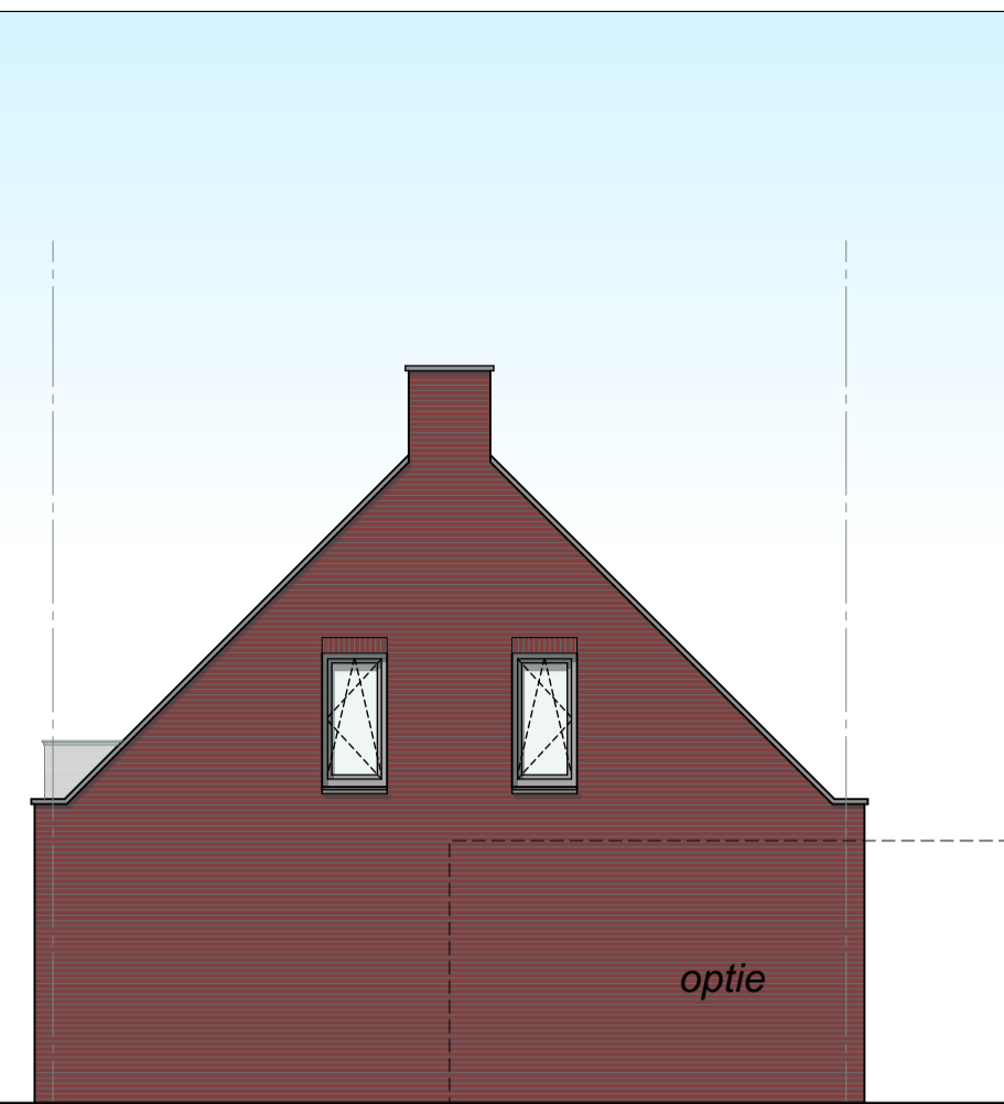
RECHTER ZIJGEVEL
