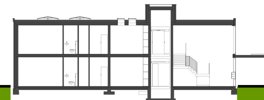
DOORSNEDE
