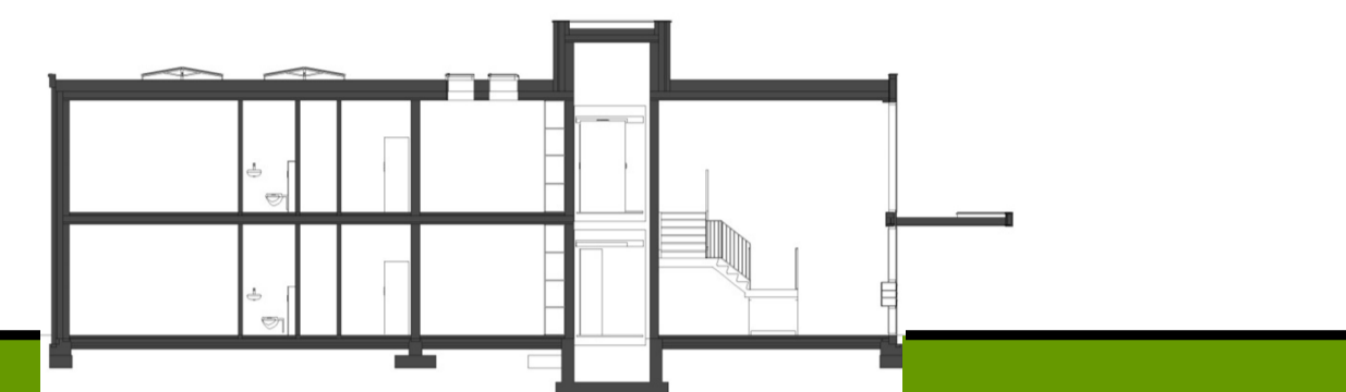
DOORSNEDE
