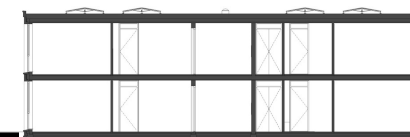
DOORSNEDE
