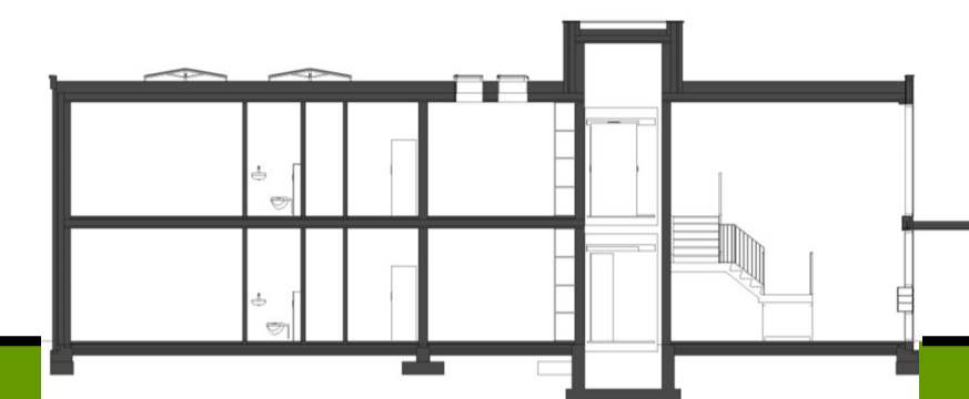
DOORSNEDE
