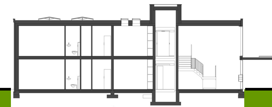
DOORSNEDE
