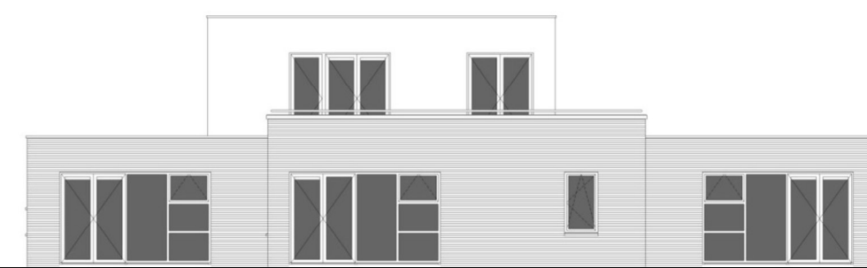
LINKER ZIJGEVEL
