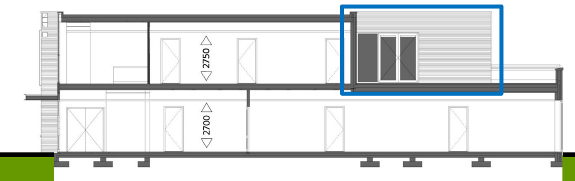
ZUIDGEVEL/ DOORSNEDE
