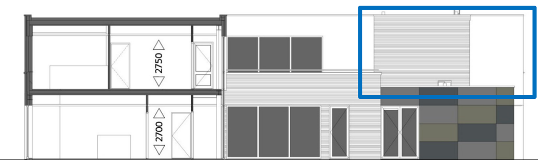
LINKER ZIJGEVEL / DOORSNEDE
